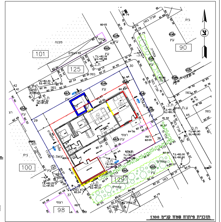
תוכנית פיתוח שטח בקנה 1:100
