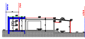
חזית א-ה בקנה 1:100
