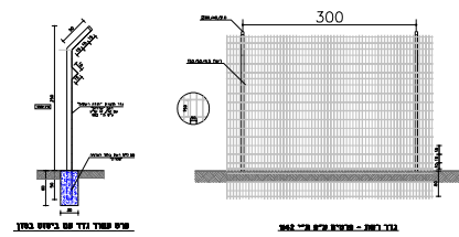
פרט שער דלת עם כניסה נגוד
