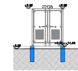
מבס צד 1100
