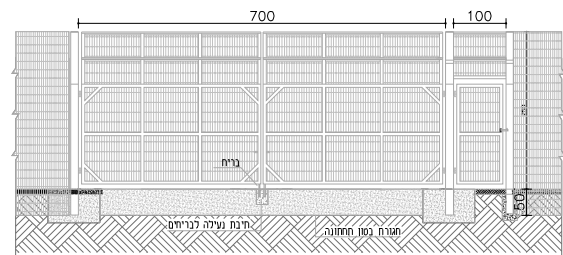
פרט שער כניסה - 1100
