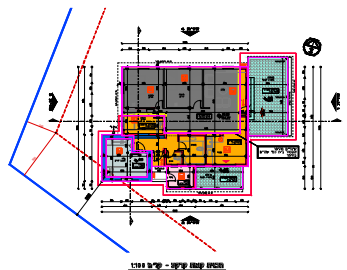
מבנה A: יחידת דיור קיימת + לגניזציות
